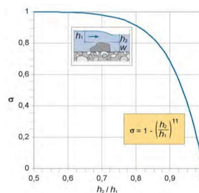
Bild 188: Rückstaubeiwert \sigma (Grafik: KRÜGER)
