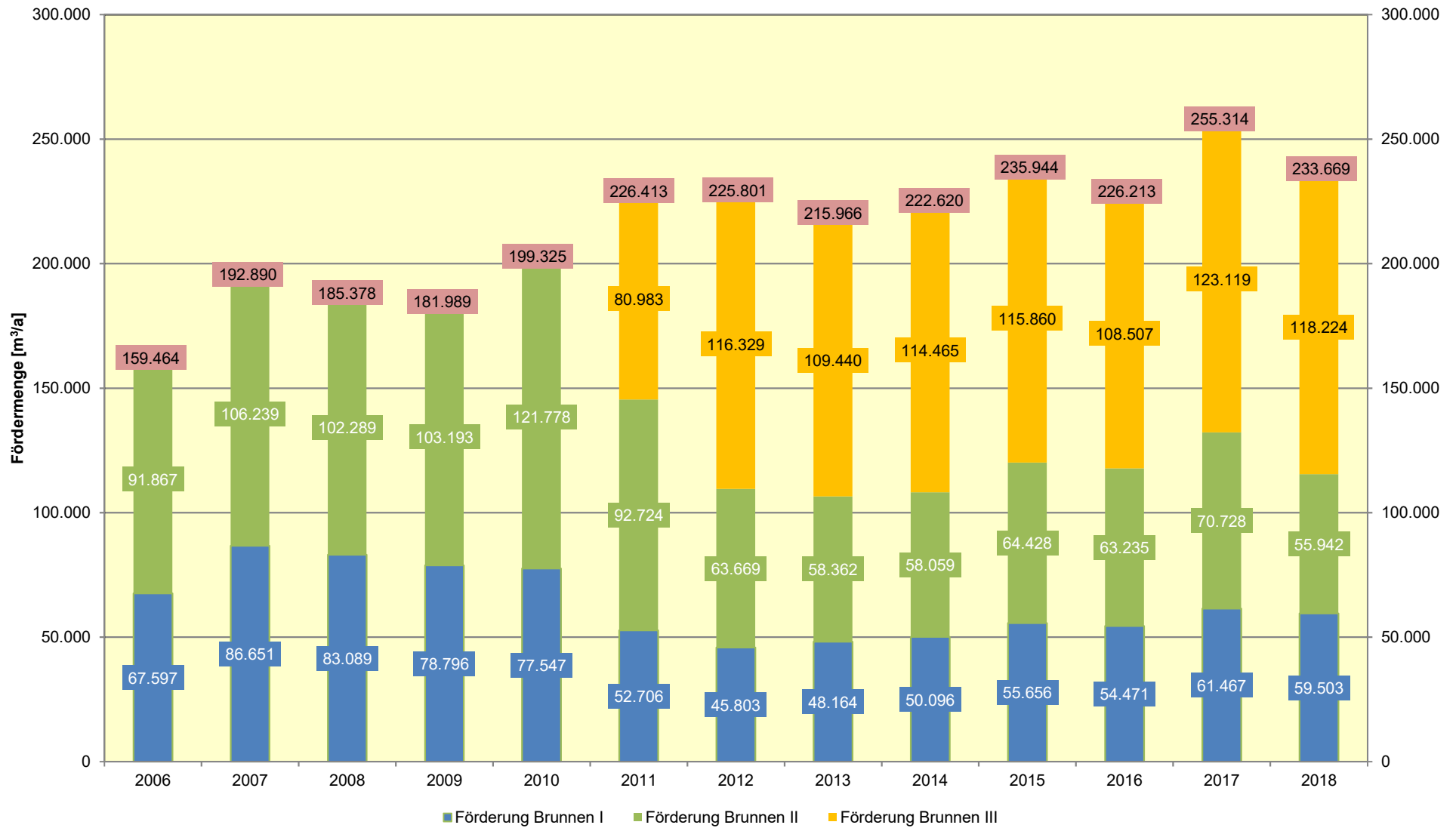
Jahresfördermengen der Brunnen Simbach I und II sowie Zollöd III, Zeitreihe 2006 bis 2018
